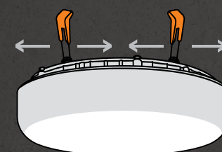
ширина монтажного отверстия от 50 до 210 мм
